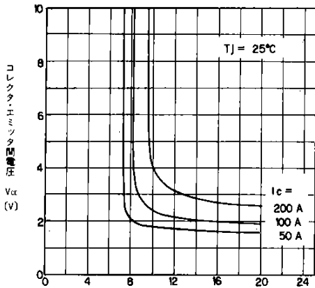
ゲート・エミッタ間電圧 V_{ge} (V) コレクタ・エミッタ間電圧—ゲート・エミッタ間電圧特性 Collector-Emittor Voltage vs. Gate-Emittor Voltage
