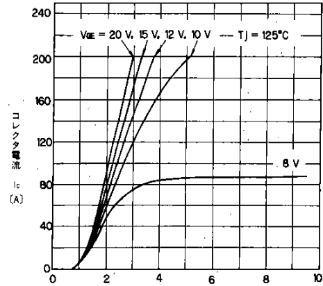
コレクタ・エミッタ間電圧 V_{ce} (V) コレクタ電流—コレクタ・エミッタ間電圧特性 Collector Current vs. Collector-Emittor Voltage
