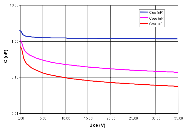
Typ. capacitances
